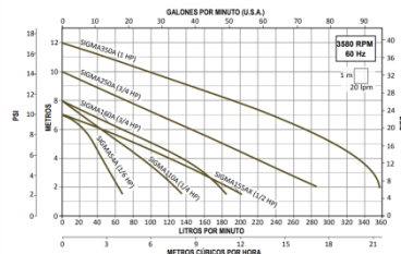
CURVAS DE OPERACIÓN
