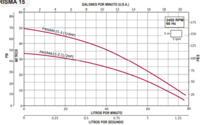
CURVAS DE OPERACIÓN PRISMA 15
