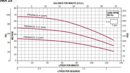
CURVAS DE OPERACIÓN PRISMA 25
